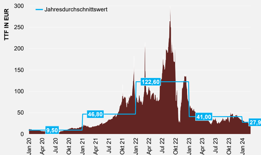
ABBILDUNG 2: ERDGASPREIS (TTF)
