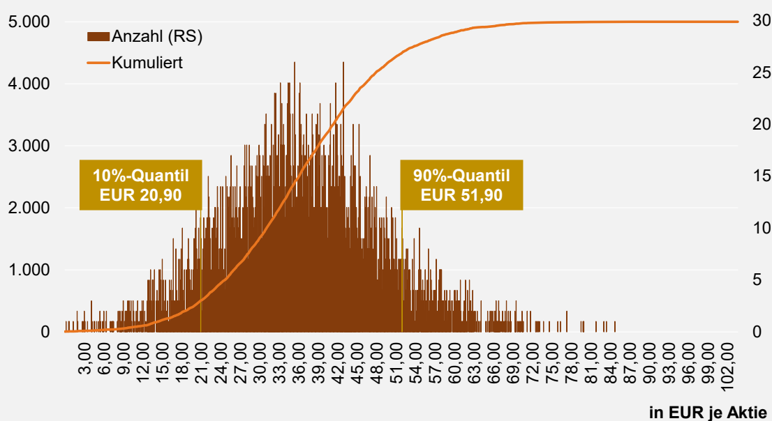
ABBILDUNG 2: MONTE-CARLO-SIMULATION (5.000 SIMULATIONEN)
